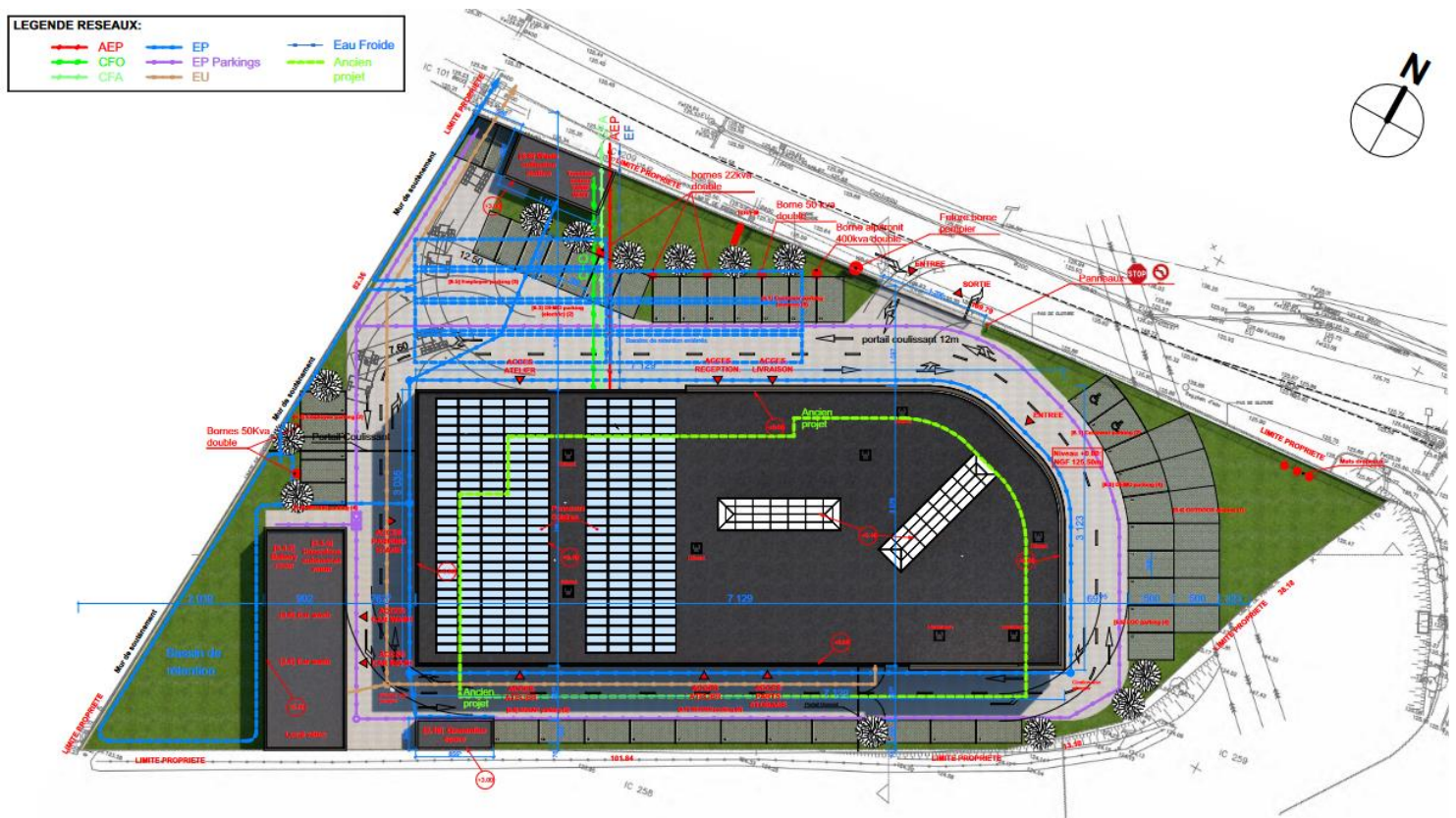
Plan masse et réseaux du projet – Source : Archipel 41
