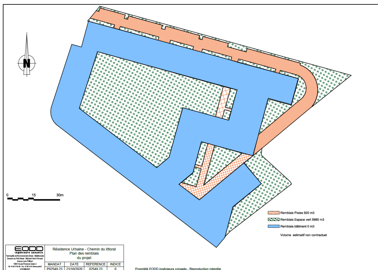
Figure 12 : Plan de localisation et volumes des remblaiements
