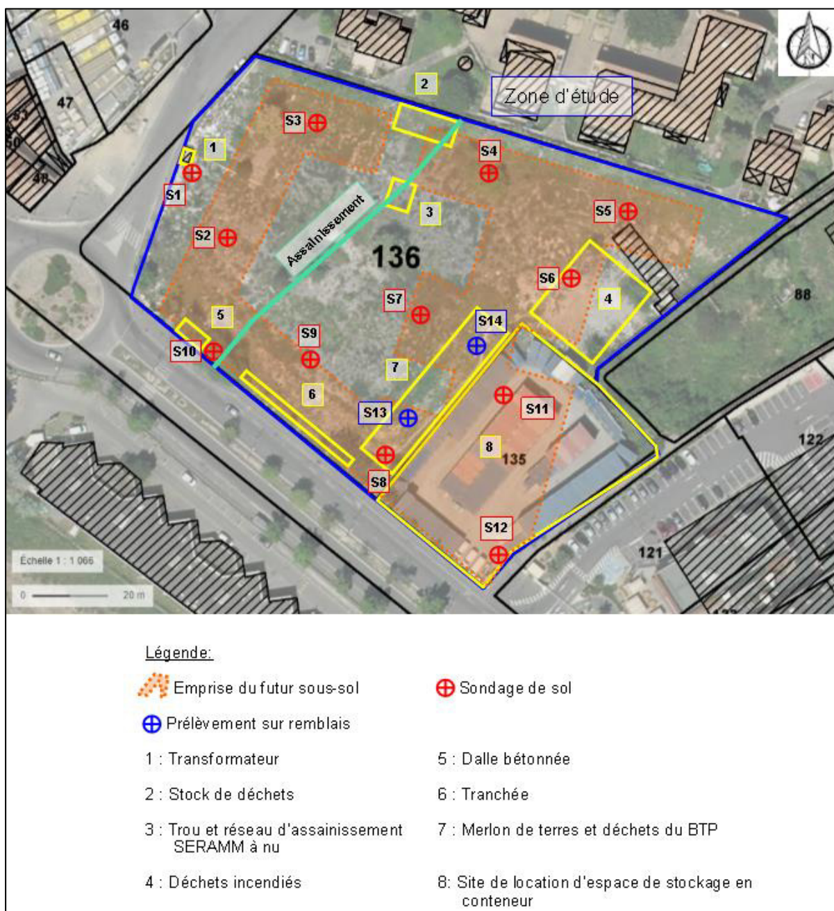
Figure 5 : Implantation des investigations réalisées sur les sols
