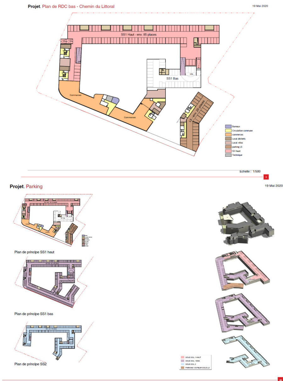
Figure 4 : Plan du RDC et parking du projet d'aménagement (source : Kaufman & Broad)
