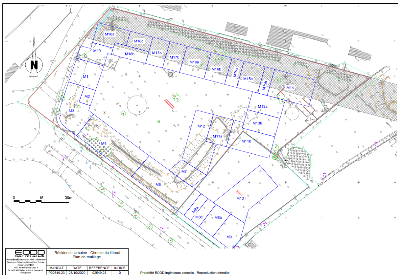
Figure 11 : Plan de maillage dimensionné en fonction des investigations
